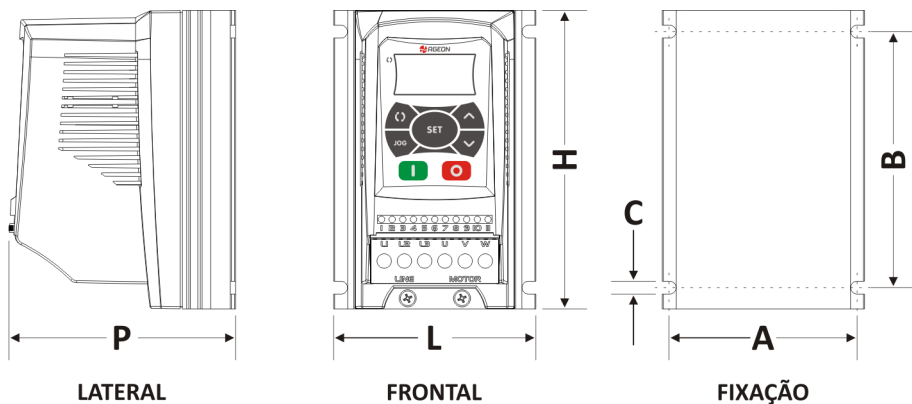
Figura 16-1 – Dimensões
